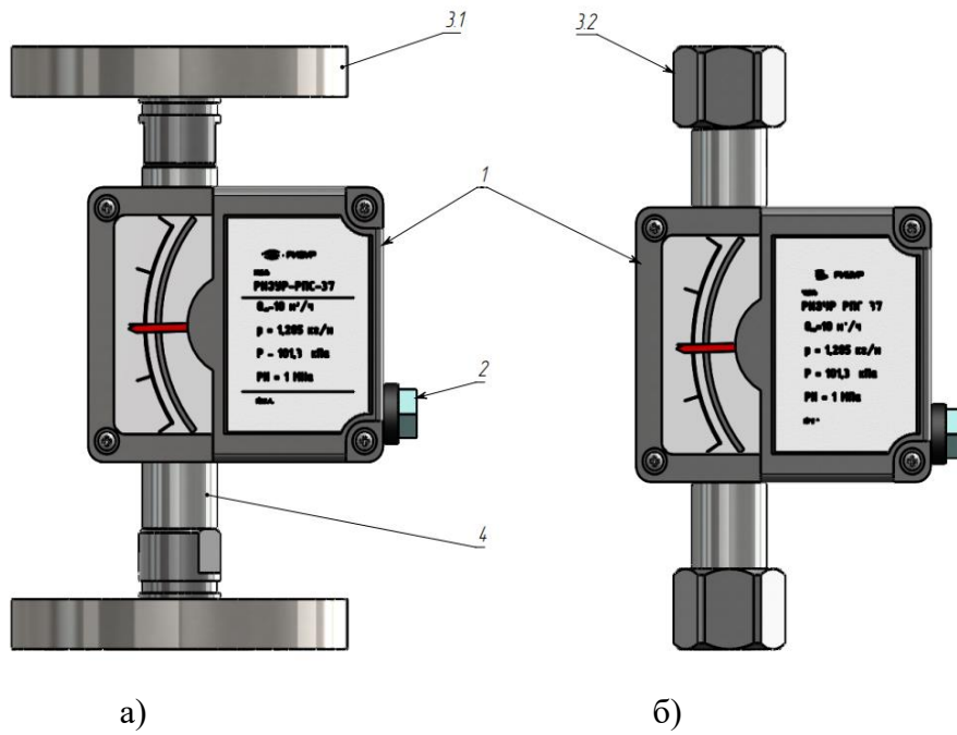
Рисунок 3 – Конструкция ротаметра фланцевого (а) и резьбового (б) типа присоединения
