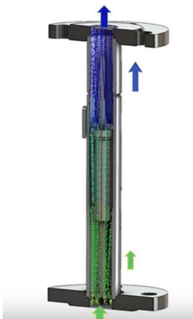
Рисунок 2 – Визуализация движения среды внутри конической трубки ротаметра.
