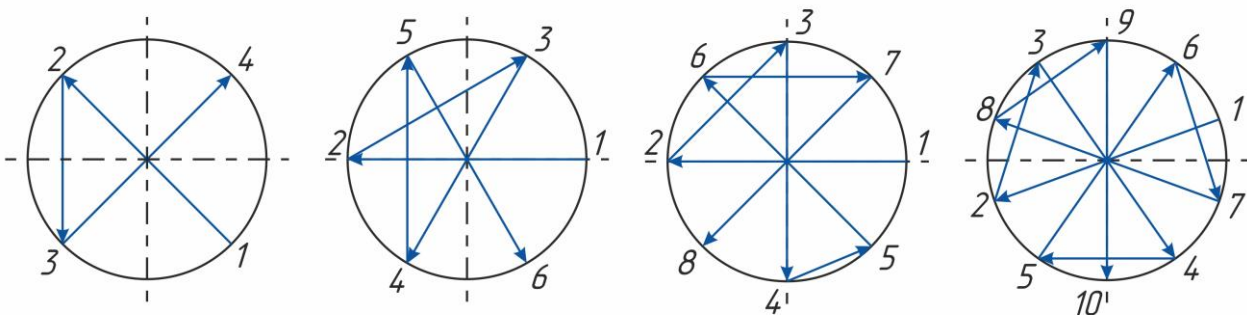
Рисунок 3. Схема затяжки фланцевых соединений
