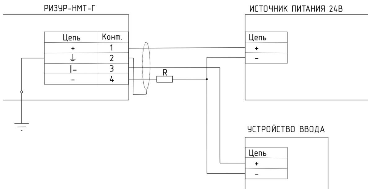
Рисунок Б.5 Схема подключения РИЗУР-НМТ-Г по токовой петле Трехпроводная схема подключения
