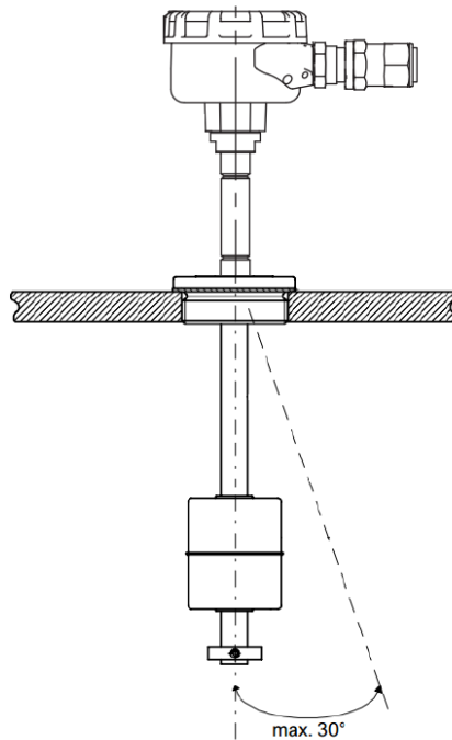
Рисунок 2. Пример монтажа уровнемера на емкости
