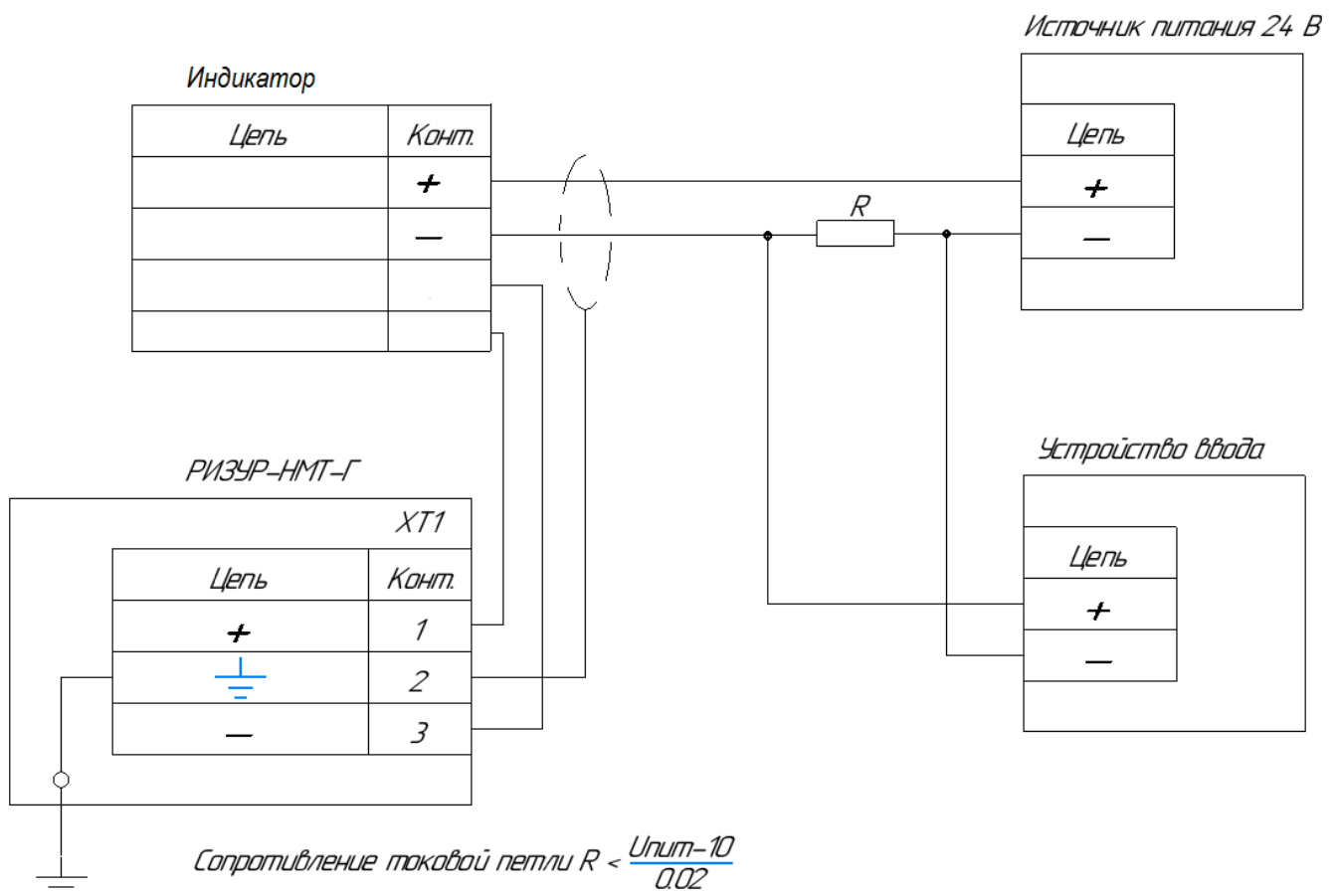
Рисунок Б.3 Схема подключения РИЗУР-НМТ-Г по токовой петле с применением барьера искрозащиты
