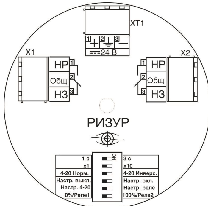
Рисункок Б.4 Внешний вид электронного блока РИЗУР-НМТ-Г двухпроводное подключение
