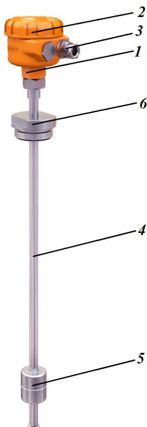
Рисунок 1. Внешний вид уровнемера поплавкового герконового РИЗУР-НМТ-Г
