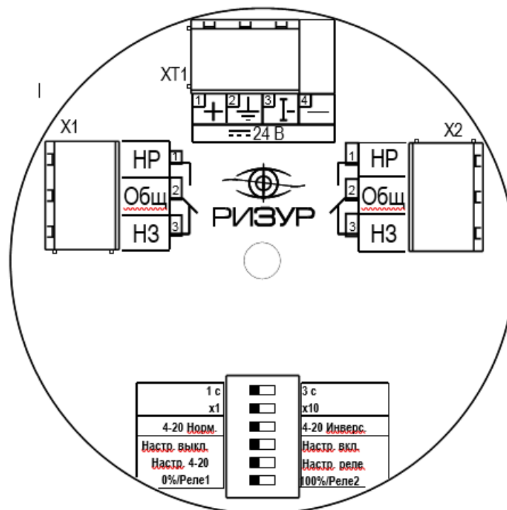
РИЗУР-НМТ-Г трехпроводное подключение
