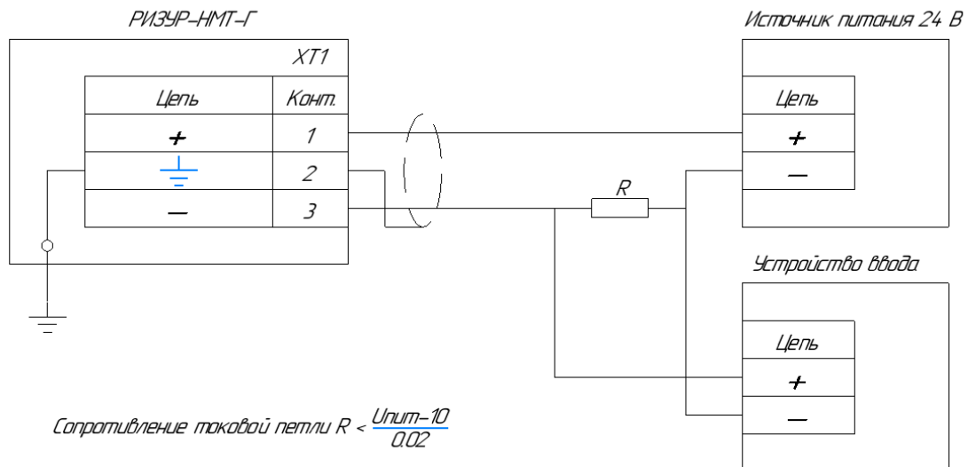
Рисунок Б.1 Схема подключения РИЗУР-НМТ-Г
