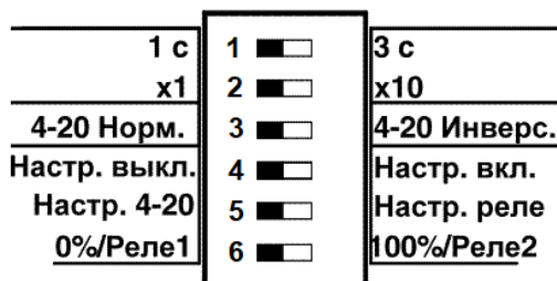
Рисунок В.1 Внешний вид группы переключателей
