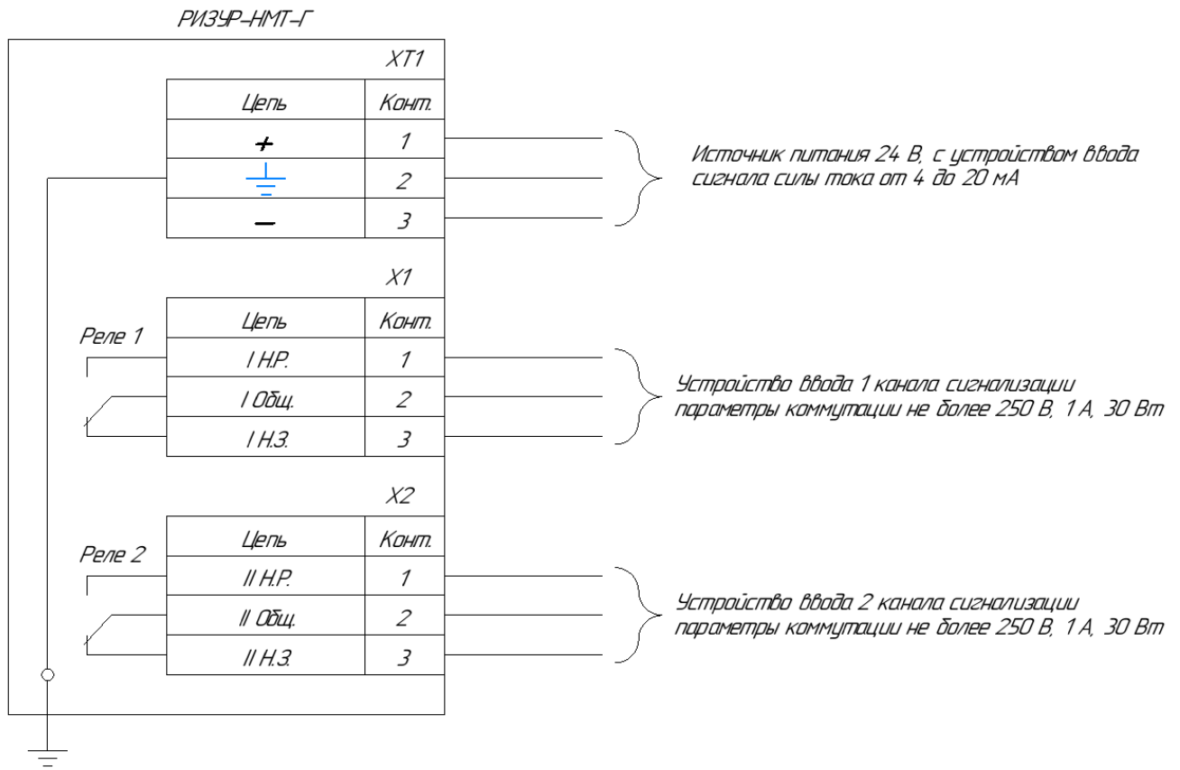
Рисунок Б.1 Схема подключения РИЗУР-НМТ-Г
