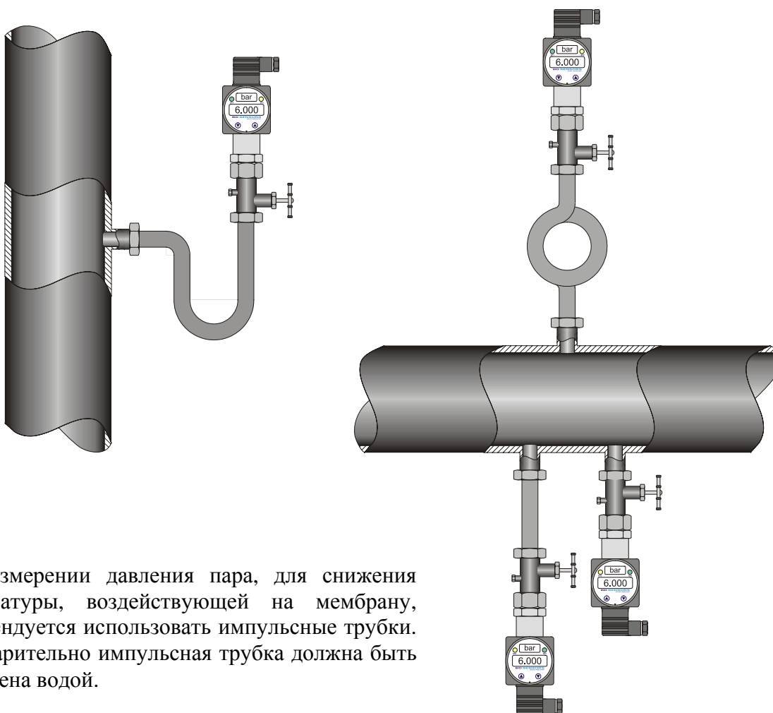
Рисунок 3. Монтаж датчика для измерения давления пара.
