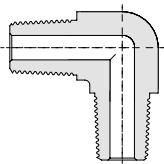
Фитинг угловой с наружными резьбами RizurLok-U-Pm-Pm
