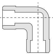
Фитинг угловой проходной под приварку внахлест RizurLok-P-W-W
