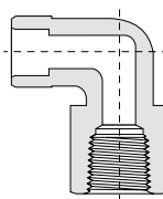
Фитинг угловой проходной под приварку внахлест с внутренней резьбой RizurLok-P-W-Pf
