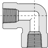
Фитинг угловой с внутренними резьбами RizurLok-U-Pf-Pf
