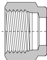
Гайка фитинга RizurLok-G
