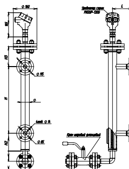
Байпасная урвнеммерная колонка РИЗУР-КБУ согласно индивидуальным требованиям заказчика
