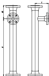
Байпасная урвнеммерная колонка РИЗУР-КБУ с креплением «бок-низ»
