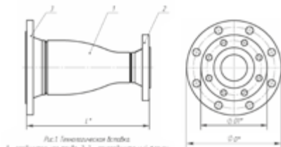
Рис.1 Технологическая вставка 1 - соединительная катушка; 2, 3 - присоединительный фланец * - соединительный диаметр для подсоединения к патрубку
