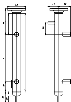
Байпасная урвнеммерная колонка РИЗУР-КБУ исполнение согласно альбому внутреннего типажа Т-ММ-04-06
