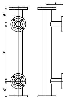
Байпасная урвнеммерная колонка РИЗУР-КБУ с креплением «бок-бок»
