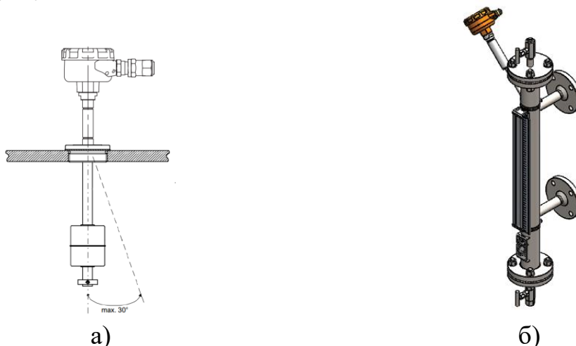
Рисунок 3 - Пример монтажа уровнемера: а) на емкости, б) на байпасной камере
