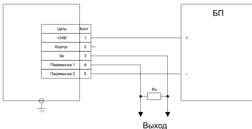
Рисунок Б.2 Схема подключения уровнемера РИЗУР-НМТ-М без взрывозащиты и со взрывозащитой вида «взрывонепроницаемая оболочка» 4х проводная схема подключения
