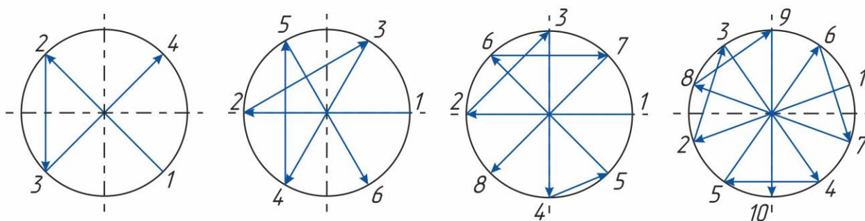
Рисунок 4 - Схема затяжки фланцевых соединений
