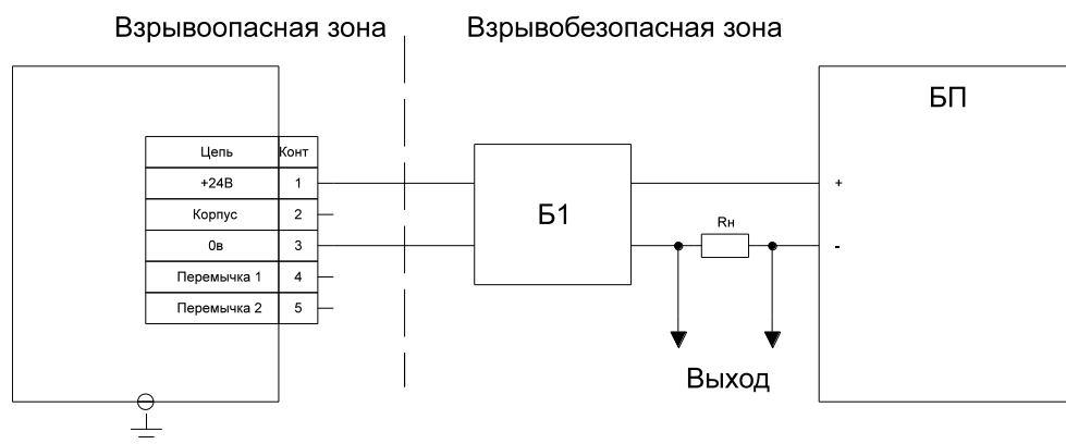
Рисунок Б.3 Схема подключения уровнемера РИЗУР-НМТ-М со взрывозащитой вида «искробезопасная цепь»
