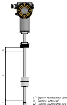
Рис. 1 – Диапазоны измерений
