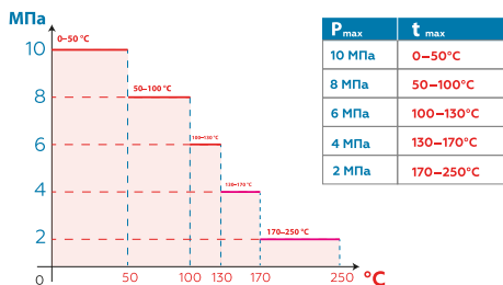
График 1 Максимальное рабочее давление в зависимости от температуры среды
