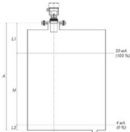
Рис. 1 - Диапазоны измерения
