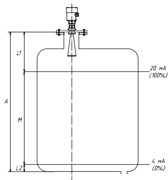
Рис. 1 - Диапазоны измерения
